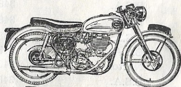
BSA 350 c.c. O.H.V. Model B 32 Gold Star 500 c.c. O.H.V. Model B 31
