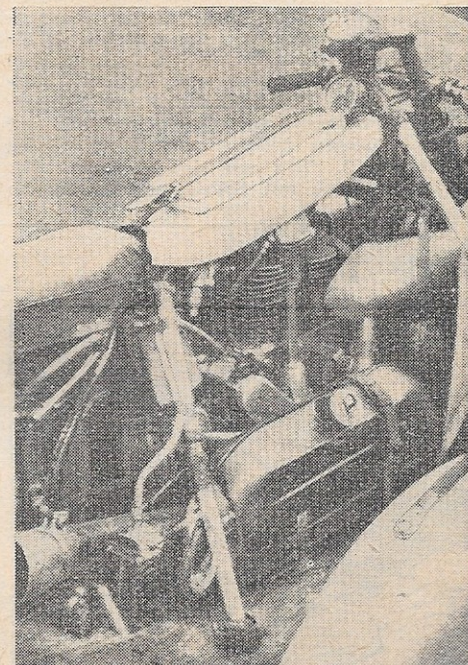
Bei dieser Norton war der Kraftstoffbehälter auf dem Seitenwagenboden befestigt. Der Kraftstoff wird bei dieser Anordnung mittels elektrischer Pumpe in die Schwimmerkammer des Vergasers gefördert Foto: Edler
